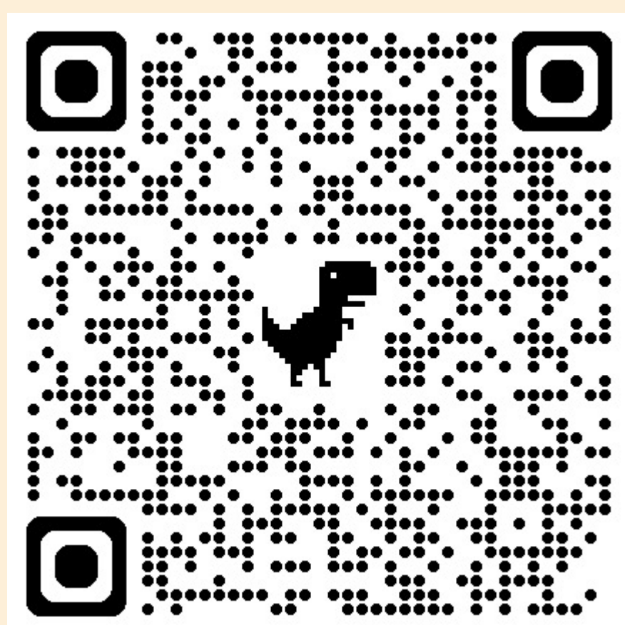
Android
