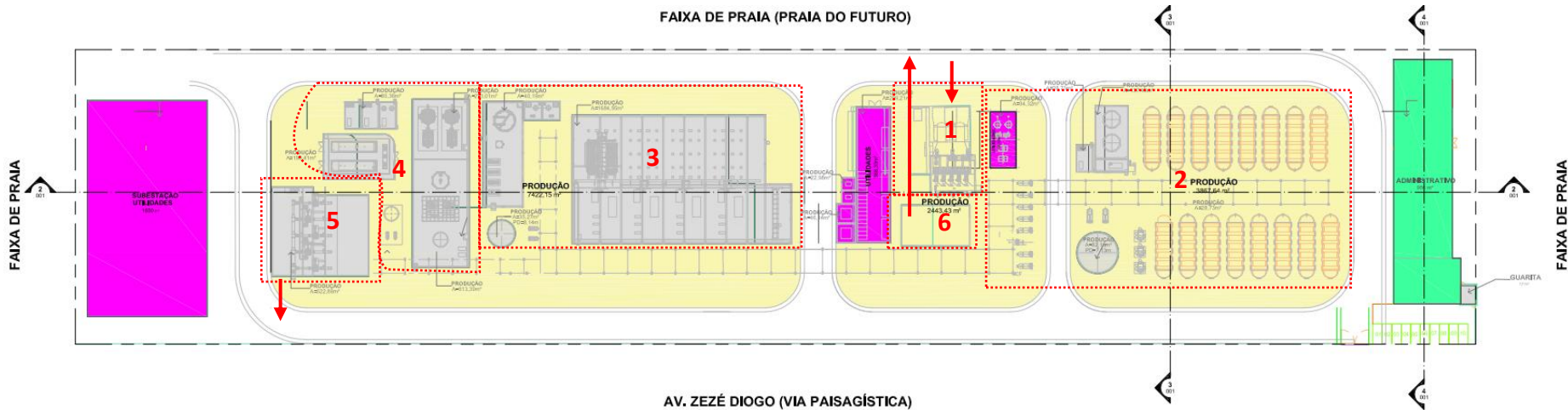
Figura 2. Layout das principais unidades componentes da planta.
