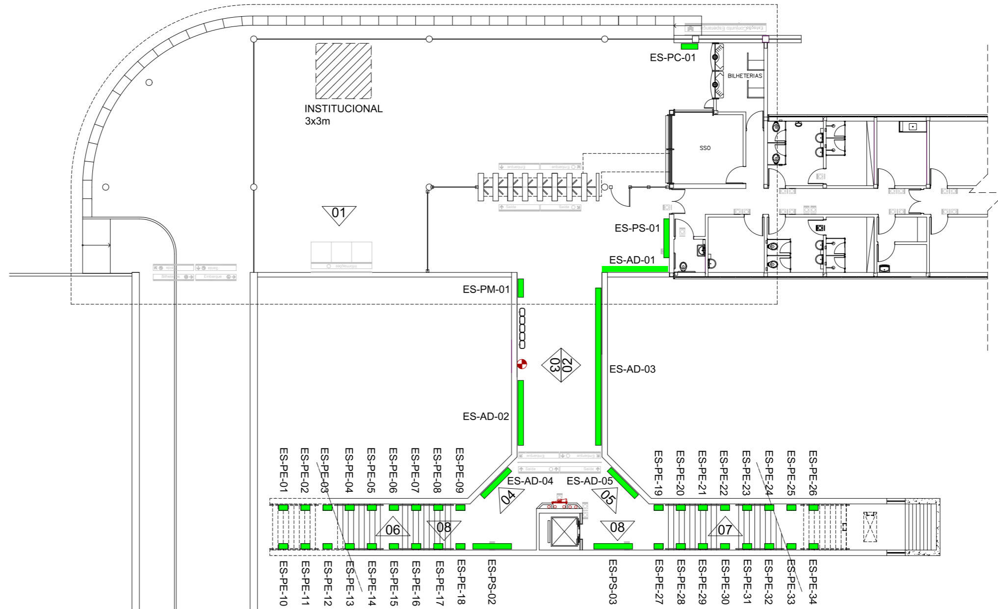
01 PLANTA BAIXA / TÉRREO ESC.: 1/20
