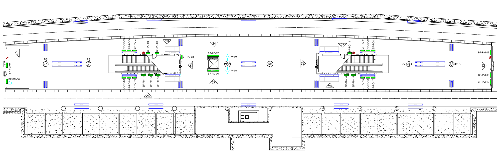
01 PLANTA BAIXA / PLATAFORMA ESC.: 1/30
