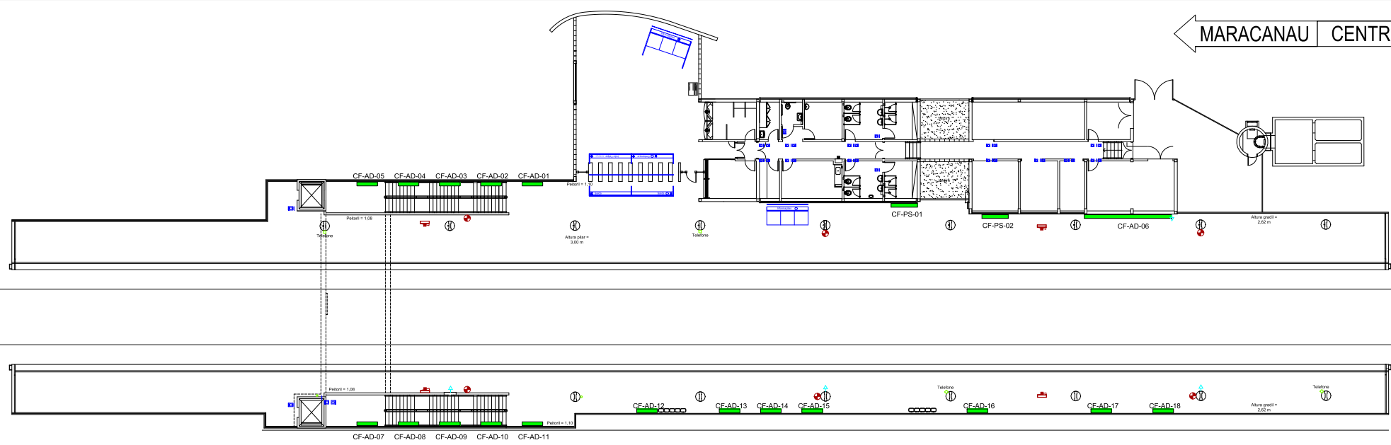
01 PLANTA BAIXA / PLATAFORMA ESC.: 1/30
