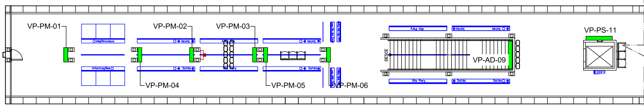
02 PLANTA BAIXA / PLATAFORMA ESC.: 1/20
