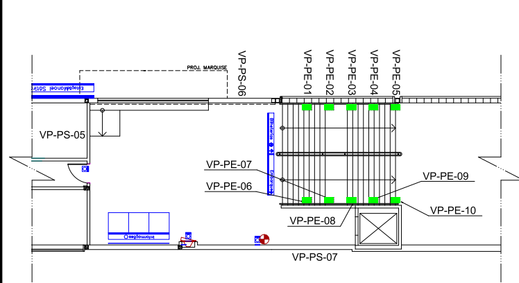
01 PLANTA BAIXA / TÉRREO ESC.: 1/20
