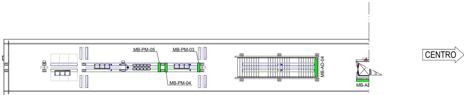
01 PLANTA BAIXA / PLATAFORMA ESC.: 1/20
