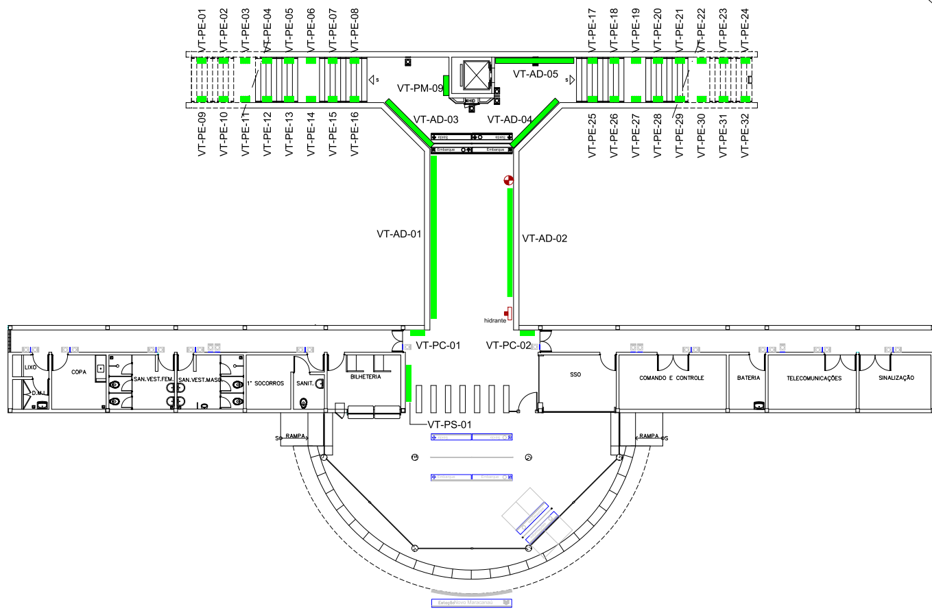
01 PLANTA BAIXA / TÉRREO ESC.: 1/20
