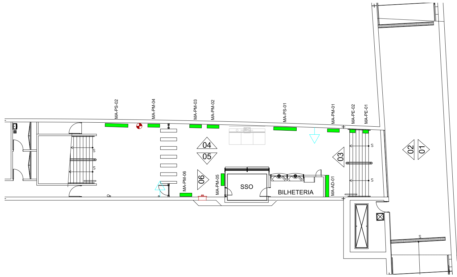
01 PLANTA BAIXA / MEZANINO ESC.: 1/15
