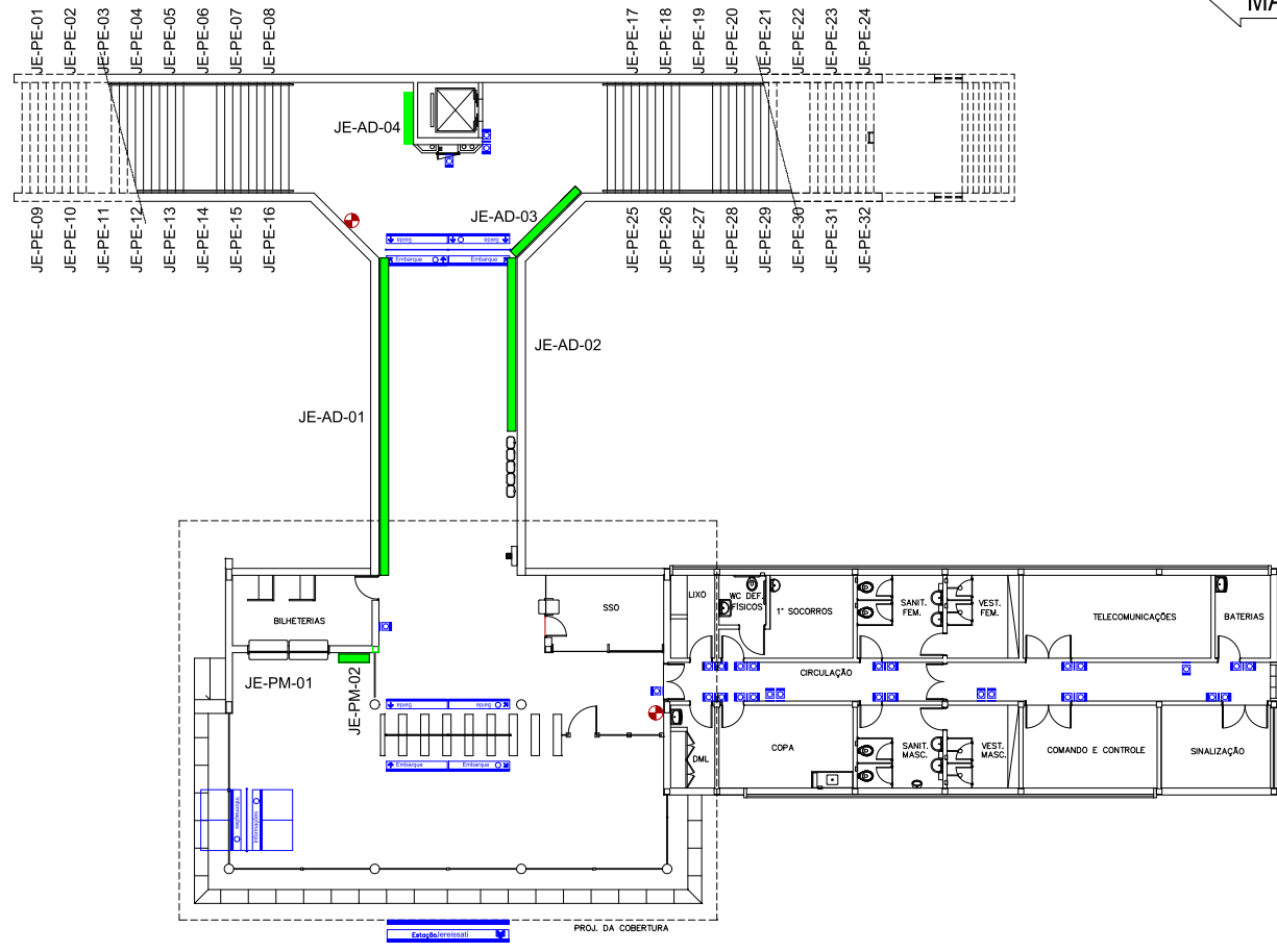
01 PLANTA BAIXA / MEZANINO ESC.: 1/20
